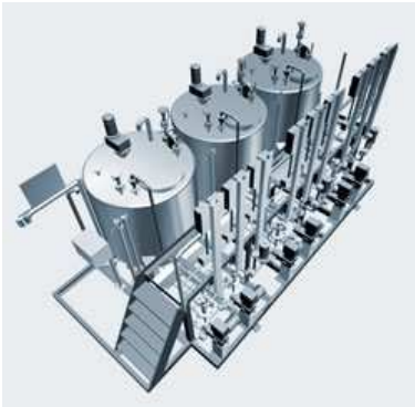
Anlagenkomponenten
